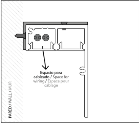
Montaje con pieza de sujeción. Pared Assembly with clamping piece. Wall
