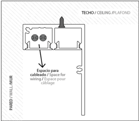
Montaje en techo Ceiling assembly
