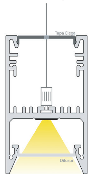
Fijación con tensor / Fixing with tensioner / Fixation avec tendeur
