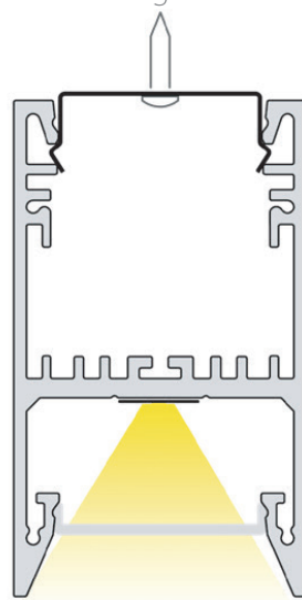
Fijación con clip / Fastener with tensioner + clip fastener / Fixation par clip
