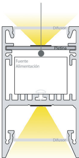
Fijación con tensor + doble difusor (up & down) / Fastener with tensioner + double diffuser (up & down) / Fixation avec tendeur + double diffuseur (haut & bas)
