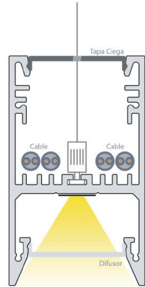
Fijación con tensor + tapa ciega / Fastener with tensioner + solid cover / Fixation avec tendeur + cache aveugle
