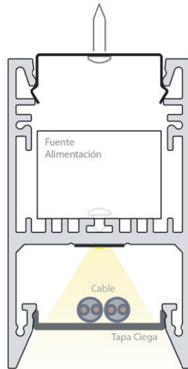
Fijación con clip + fuente alimentación + cableado / Clip fastener + power supply + cabling / Clip de fixation + alimentation + câblage
