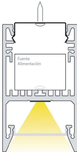
Fijación con clip + fuente alimentación / Clip fastener + power supply / Clip de fixation + alimentation
