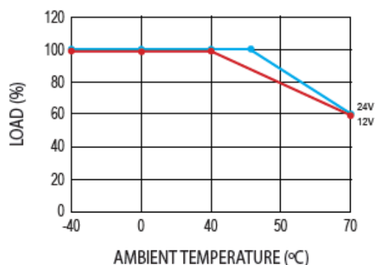
Potencia de salida - Temperatura
